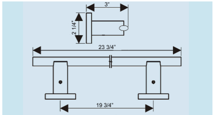
164/59 Nerea Towel Bar
